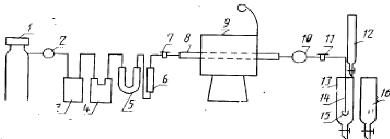
Схема установки для определения серы титриметрическим методом
